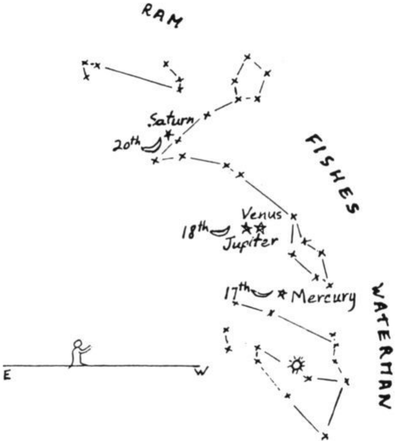
De westelijke hemel bij zonsondergang op 23 februari 1999 en de posities van de maan op 17,18 en 20 februari.
